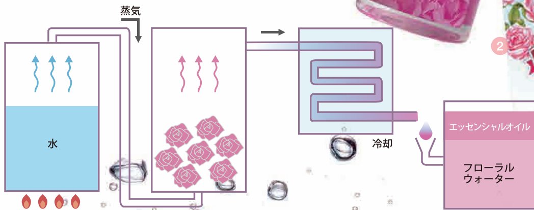
図：精油の水蒸気蒸留法
